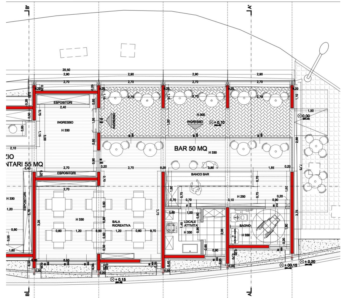
DETTAGLIO ARREDI BAR
